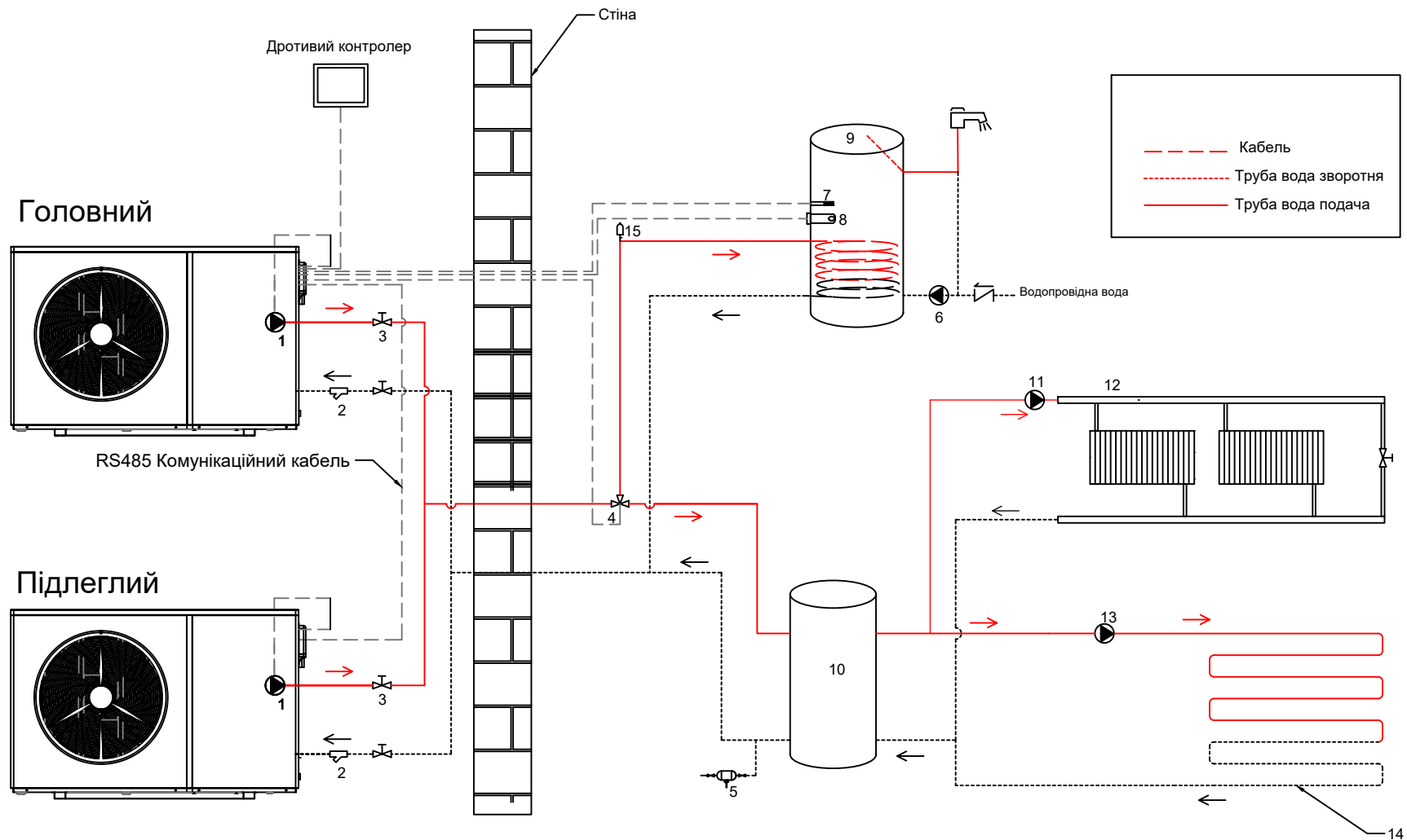
Опалення & Охолодження + Гаряча вода. Монтажна схема.
