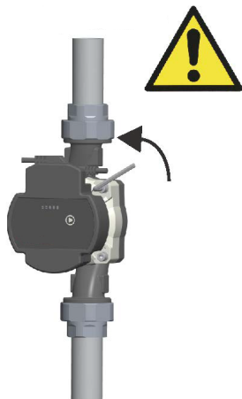
4) Зніміть шестигранні болти за допомогою шестигранного ключа
